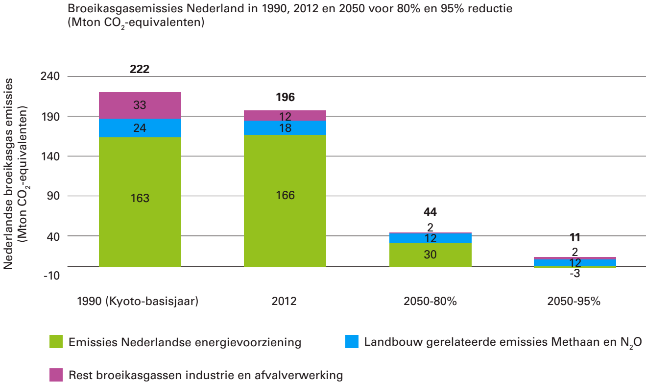
Figuur 4-1: Broeikasgasemissies (Mt CO 2 -equivalenten) voor de energievoorziening in 1990 en 2050
